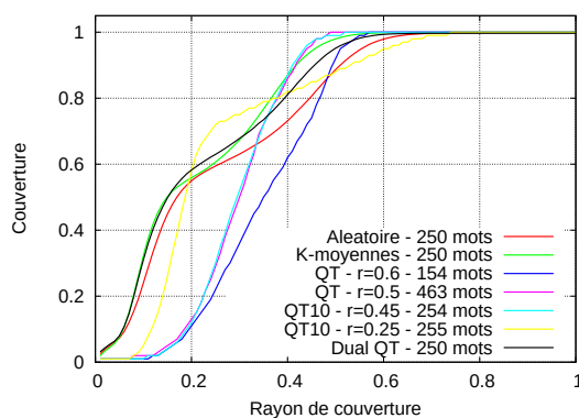
FIG. 3.8 – Pascal VOC 2007, descripteurs fou16 et eoh16, couverture des vocabulaires de taille 250
