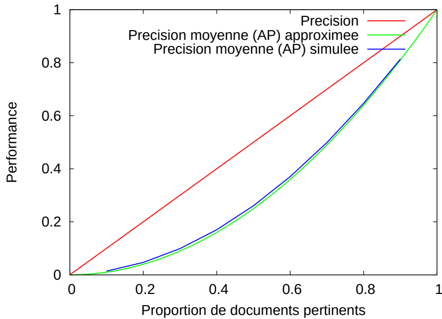
FIG. 2.4 – Evolution de la précision et de la précision moyenne en fonction de la proportion de documents pertinents pour un classement aléatoire.
