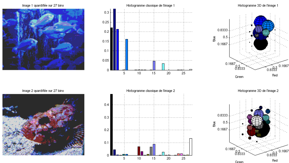
FIG. 2.2 – Histogrammes RGB de deux images
