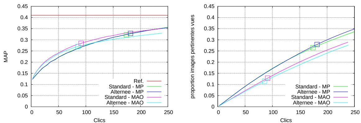
FIG. 3.38 – Pascal VOC 2007, bouclage de pertinence, simulation de l'utilisateur EQU, performances en fonction du nombre de clics
