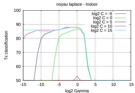
FIG. 2.31 – ImagEVAL-5, optimisation du noyau laplace, Indoor
