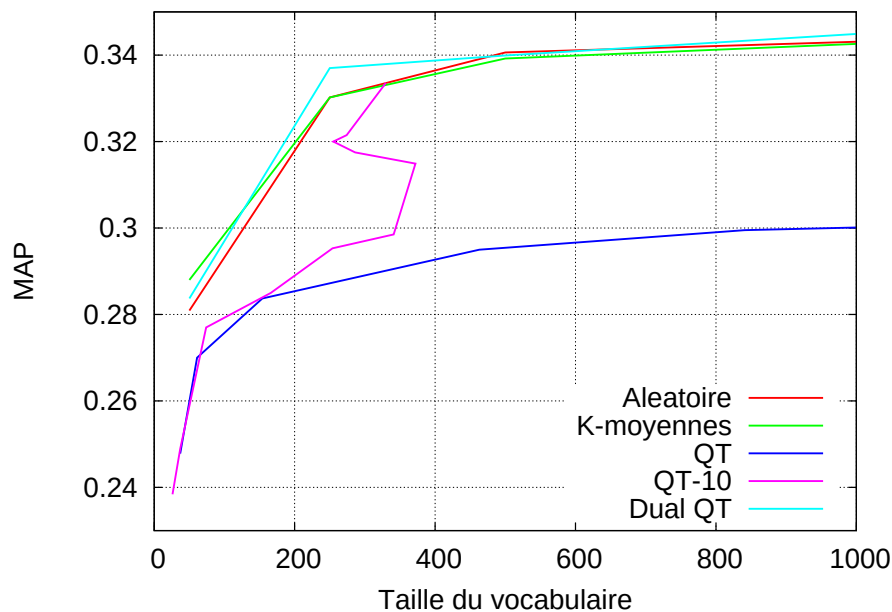
FIG. 3.10 – Pascal VOC 2007, descripteurs fou16 et eoh16, performance selon les algorithmes de partitionnement
