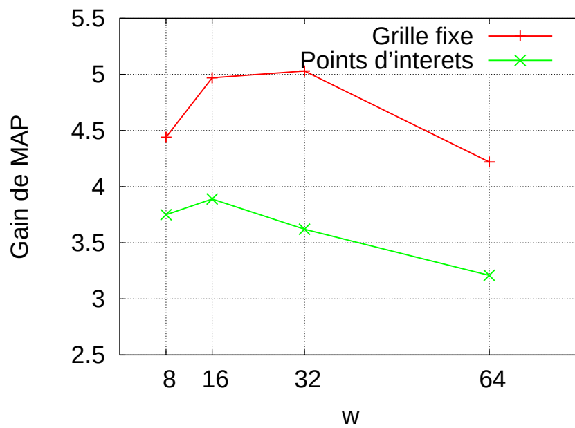
FIG. 3.22 – ImageEVAL-4, gain de MAP moyen selon la taille de la fenêtre par rapport aux résultats de référence
