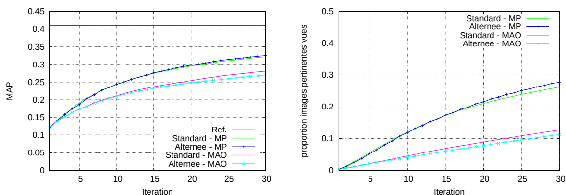
FIG. 3.33 – Pascal VOC 2007, bouclage de pertinence, simulation de l'utilisateur EQU
