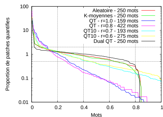
FIG. 3.12 – Pascal VOC 2007, descripteur prob64, quantification des vocabulaires de taille 250
