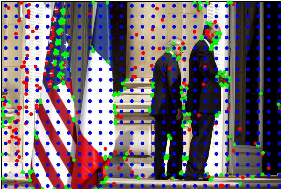
FIG. 3.23 – ImageEVAL-4, localisation des patches SIFT (rouge), Harris (vert) et grille fixe (bleu). ©Bassignac-Gamma.
