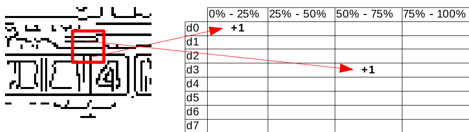
FIG. 2.23 – Fonctionnement du descripteur LEOH
